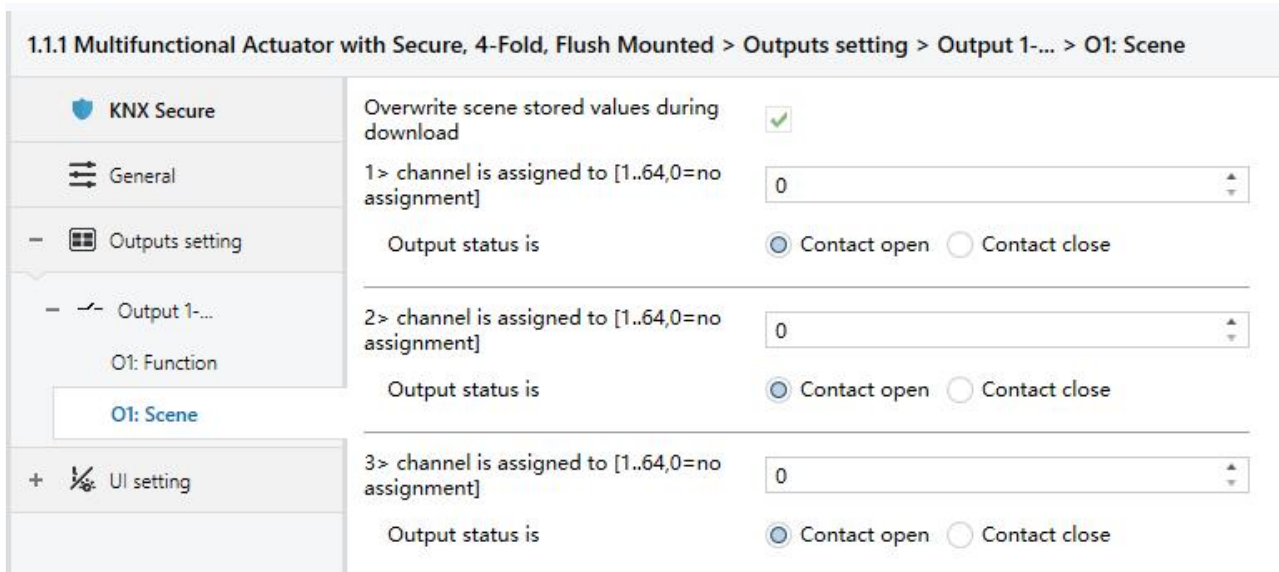
图 4.4.4 参数设置界面 “Output X: Scene”
