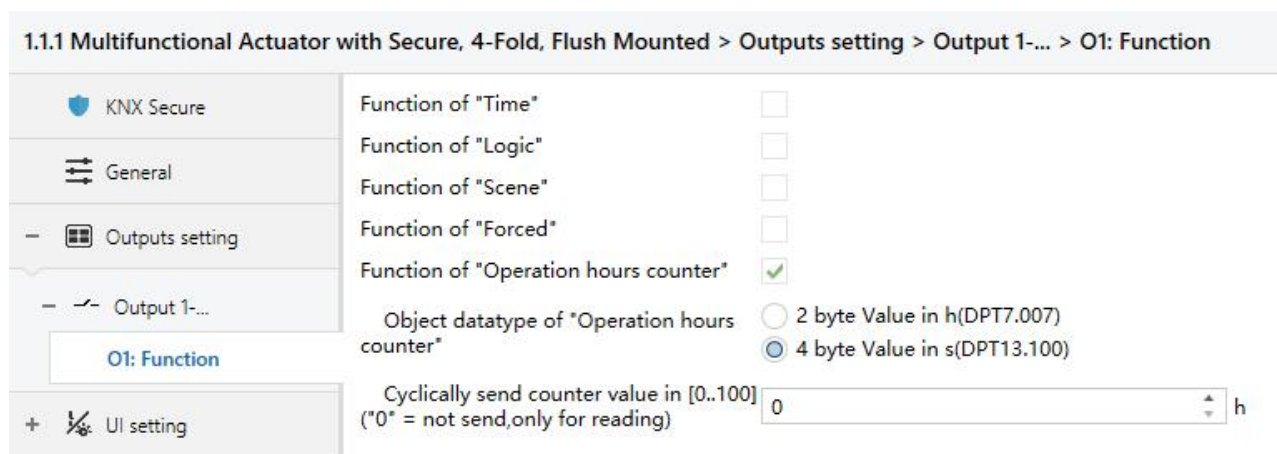
图 4.4.6 参数设置界面 “Output X: Operation hours counter”
