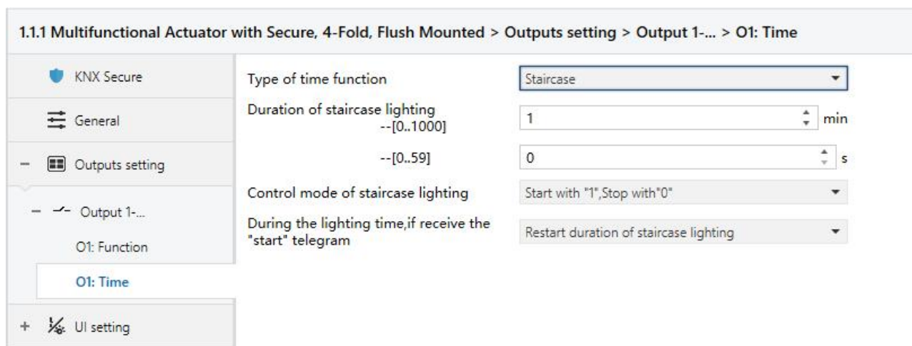
图 4.4.2.3 参数设置界面 “Output X: Time - Staircase”
