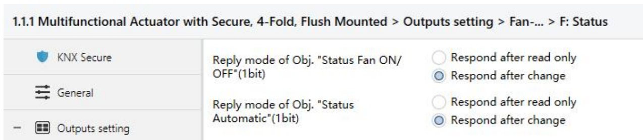
图 4.8.1.2· 参数设置界面 “Fan: Status”
