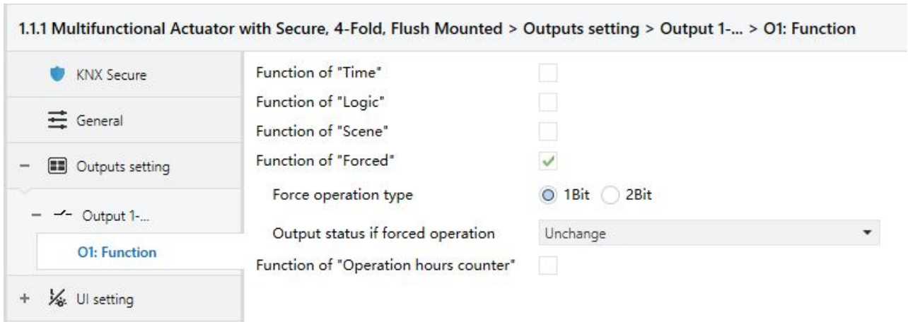
图 4.4.5 参数设置界面 “Output X: Forced”
